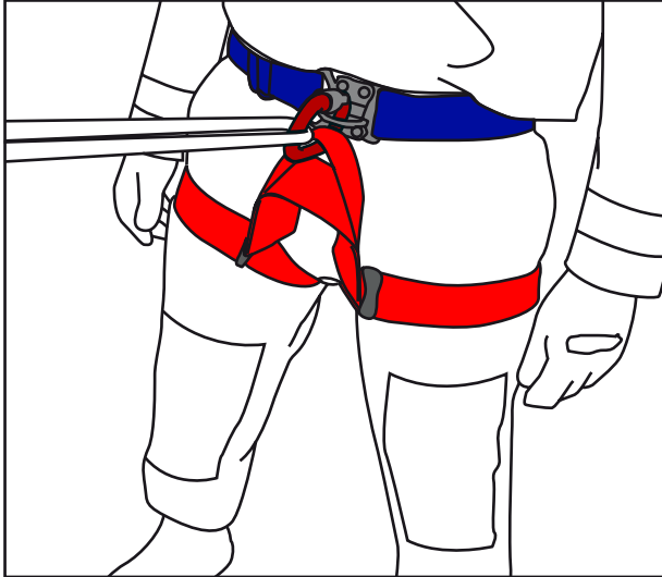
Auto évacuation d'urgence: la ceinture C-DROP + la sangle S-DROP rassemblés par un mousqueton, deviennent un baudrier permettant une évacuation d'urgence.
